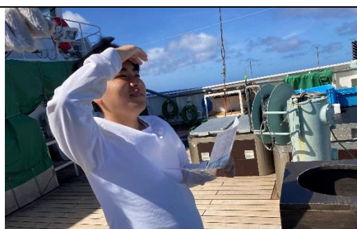
海洋観測 (雲量・雲形)
