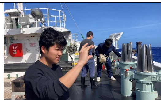
海洋観測 (水色)
