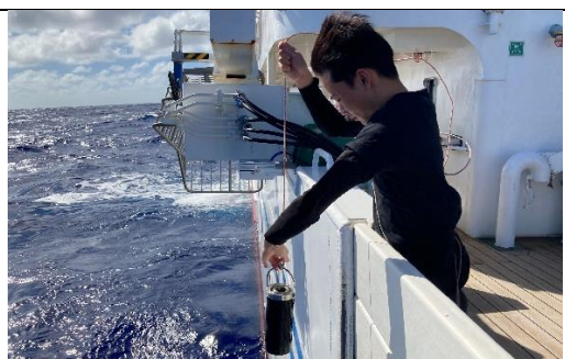
海洋観測 (海水表面温度)
